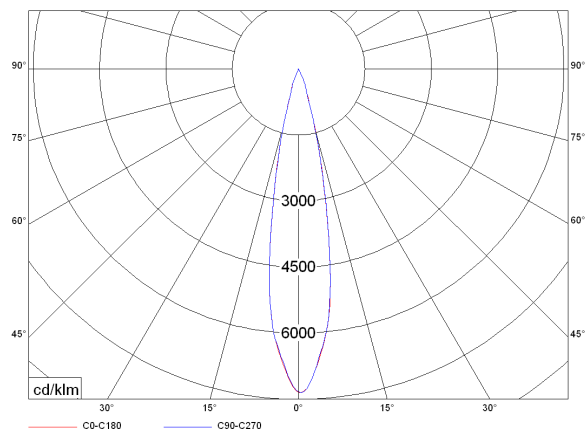
LEDspot111 50 adv 830
