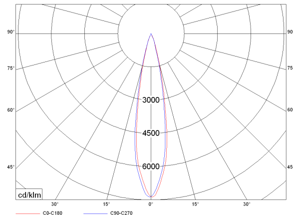
LEDspot111 50 adv 827
